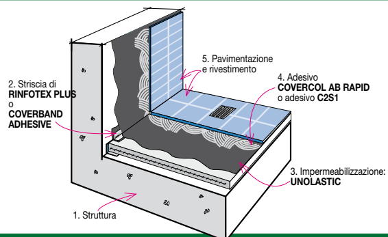
Con UNOLASTIC si possono impermeabilizzare bagni e docce senza l'utilizzo di armature
