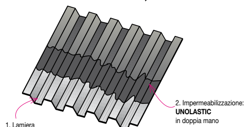
UNOLASTIC può essere sovraverniciato con la pittura riflettente WHITE REFLEX o con la pittura ELASTOLIQUID S
